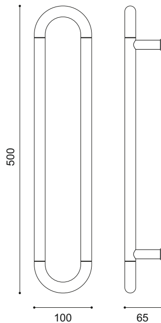
FF.TUBA.PULL.PB. 500
