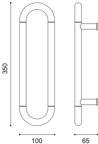
FF.TUBA.PULL.PB. 350
