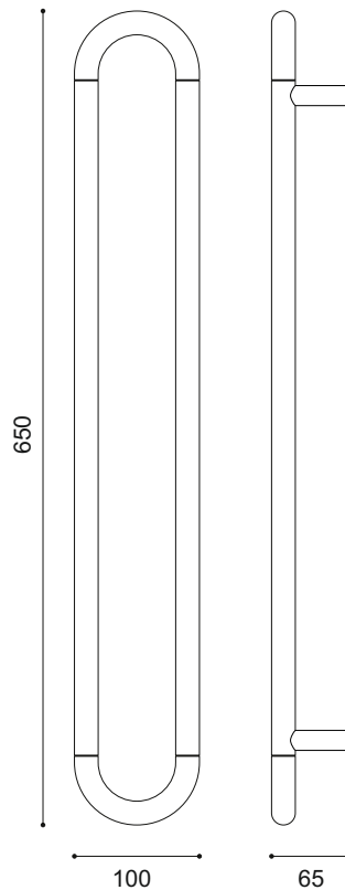
FF.TUBA.PULL.PB. 650
